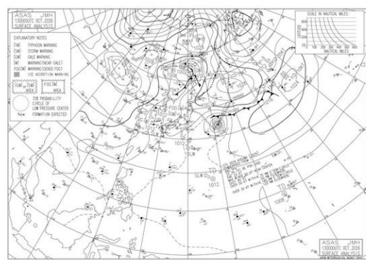
ASAS 24時間前 10月13日 9時
